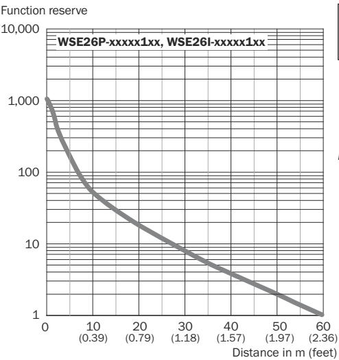
Рисунок 68: Характеристика 1
