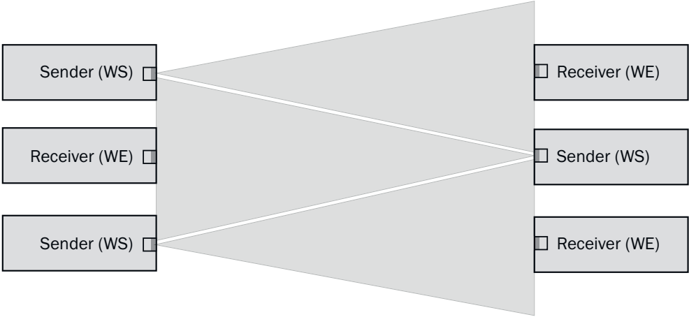
插图 73: 多个对射式光电传感器的布置
