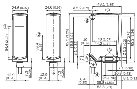
Figura 63: Desenho dimensional 1, cabo
