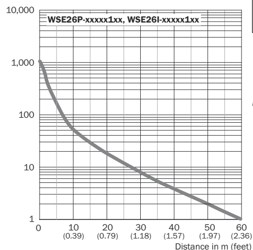
Figura 20: Curva característica 1
