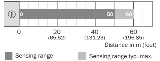
Figura 37: Diagramma a barre 1
