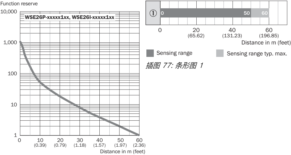
插图 76: 特征曲线 1
