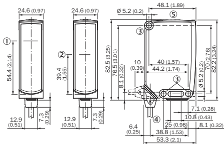
Figura 39: Disegni dimensionali 1, cavo
