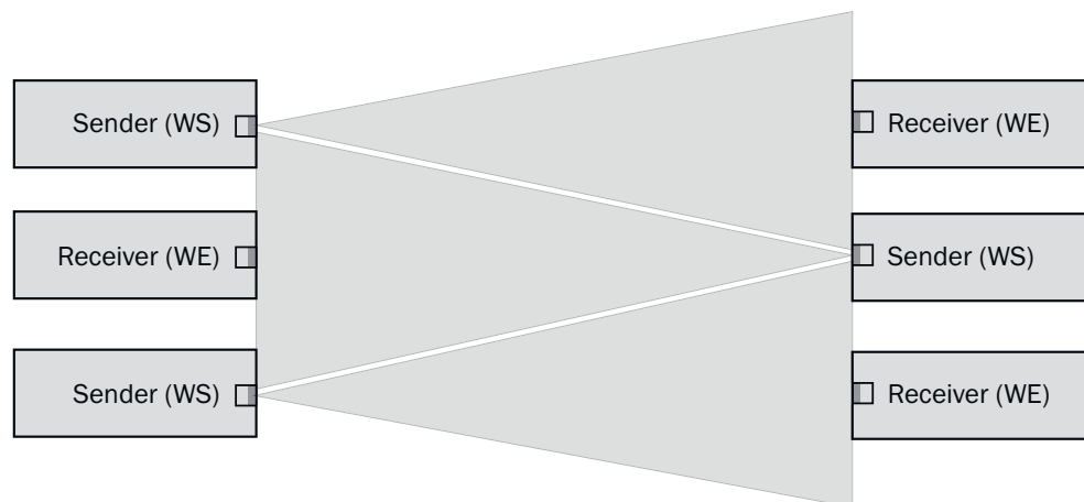
Figura 57: Disposição de várias barreiras de luz unidirecionais
