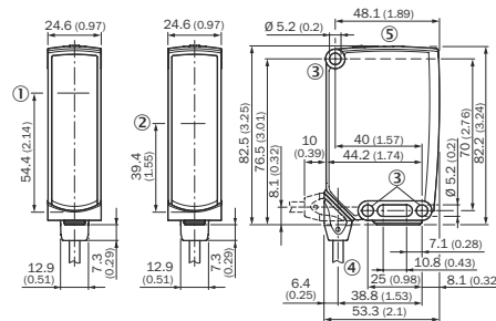
Rysunek 55: Rysunek wymiarowy 1, przewód
