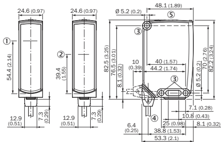
插图 79: 尺寸图 1, 电缆
