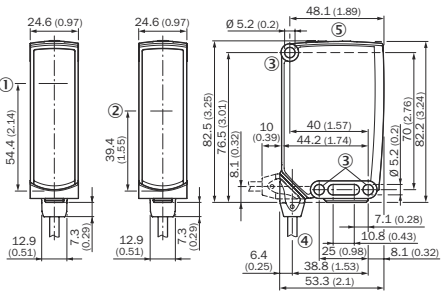
Figura 23: Dibujo acotado 1, cable
