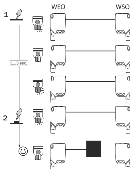
Рисунок 70: WSE26x-xxxxxx3xAxx, настройка расстояния срабатывания с помощью кнопки обучения
