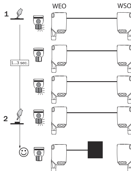
Abbildung 6: WSE26x-xxxxxx3xAxx, Einstellung des Schaltabstands mit Teach-in-Taste
