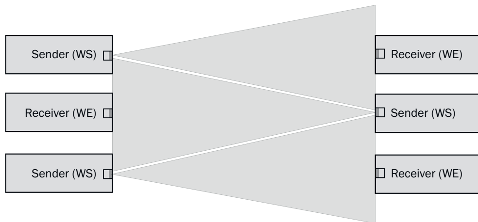
Rysunek 49: Rozmieszczenie wielu fotoprzełączników barierowych
