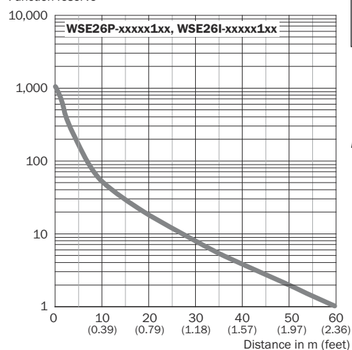
Figura 60: Curva característica 1
