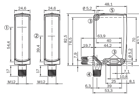
Abbildung 8: Maßzeichnung 2, Stecker
