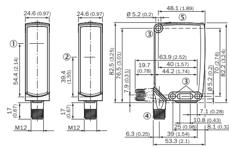
図 48: 寸法図 2、オスコネクタ
