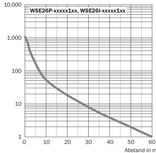
Abbildung 4: Kennlinie 1
