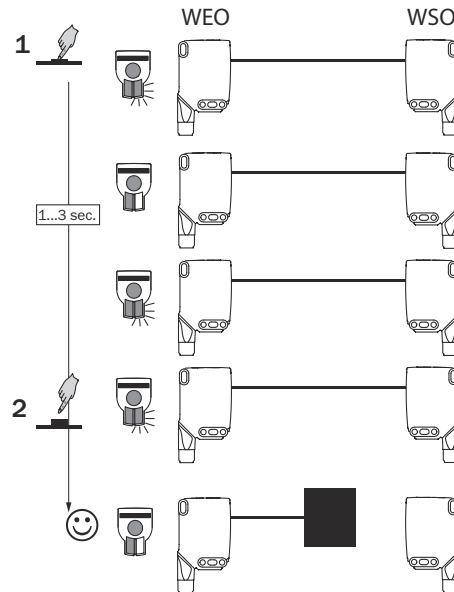
Figura 38: WSE26x-xxxxxx3xAxx, impostazione della distanza di lavoro con pulsante teach-in
