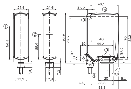
Abbildung 7: Maßzeichnung 1, Leitung
