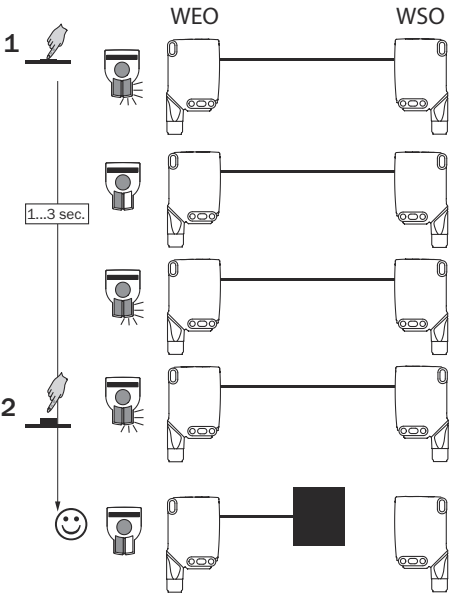
插图 78: WSE26x-xxxxxx3xAxx, 通过示教键调整触发感应距离
