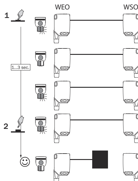
Illustration 30: WSE26-xxxxxx3xAxx, réglage de la distance de commutation avec le bouton d'apprentissage
