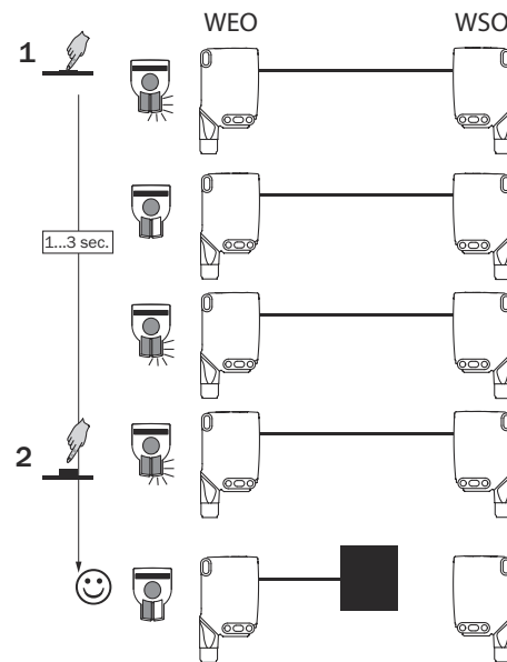
Figura 22: WSE26x-xxxxxx3xAxx, ajuste de la distancia de conmutación con una tecla teach-in
