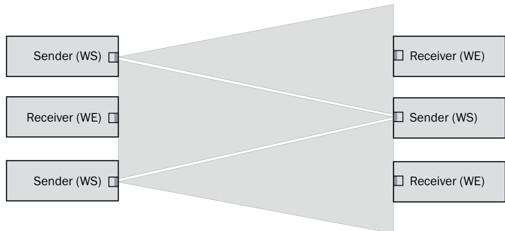
図 41: 複数の透過形光電センサの配置
