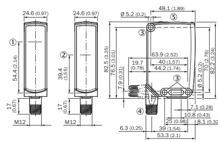
Рисунок 72: Масштабный чертёж 2, штекер
