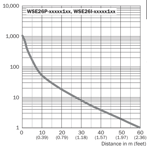
図 44: 特性曲線 1
