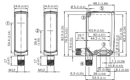
Rysunek 56: Rysunek wymiarowy 2, wtyk
