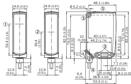
Illustration 31: Plan coté 1, câble
