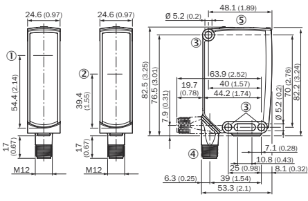
Figura 24: Dibujo acotado 2, conector macho
