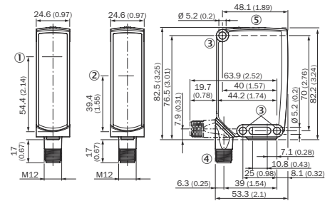
Illustration 32: Plan coté 2, connecteur mâle
