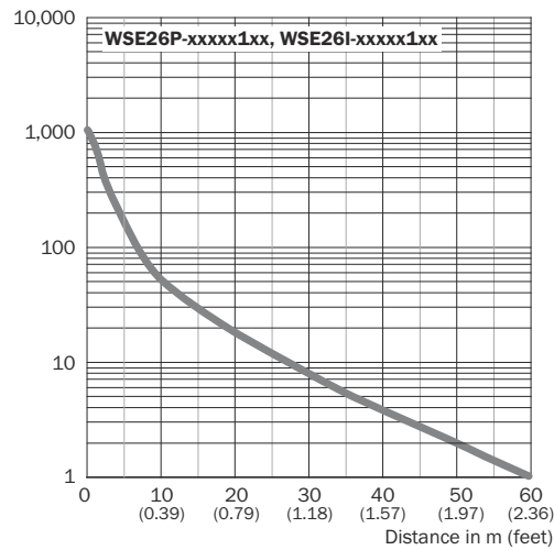
Figura 36: Linea caratteristica 1
