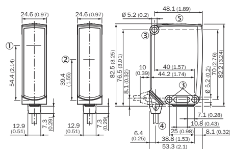
Рисунок 71: Масштабный чертёж 1, кабель
