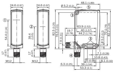
插图 80: 尺寸图 2, 插头
