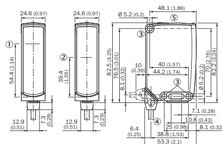
図 47: 寸法図 1、ケーブル
