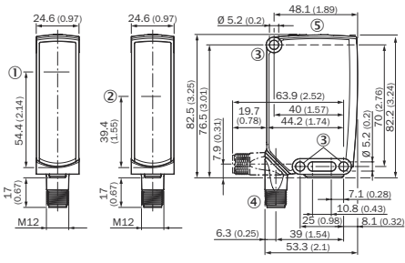
Figura 40: Disegni dimensionali 2, connettore maschio
