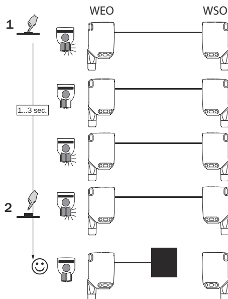
図 46: WSE26x-xxxxxx3xAxx、ティーチンボタンによる検出距離の設定
